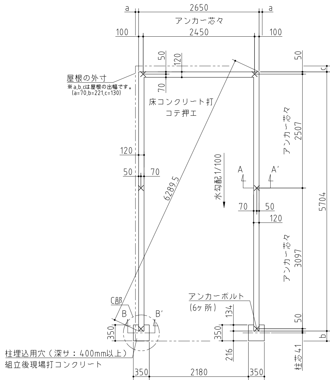
基礎詳細図 S=1/20
